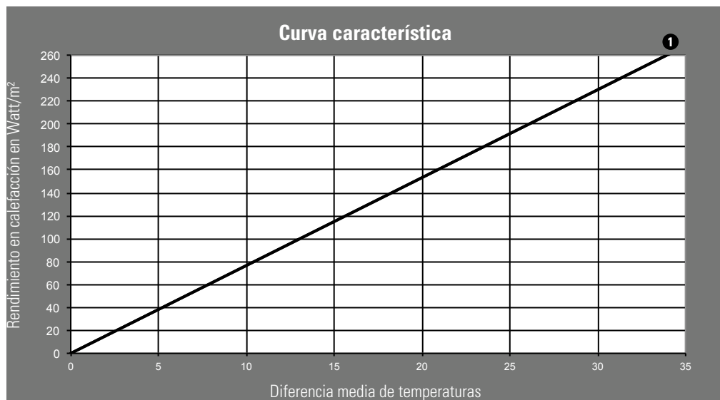
Curva característica
