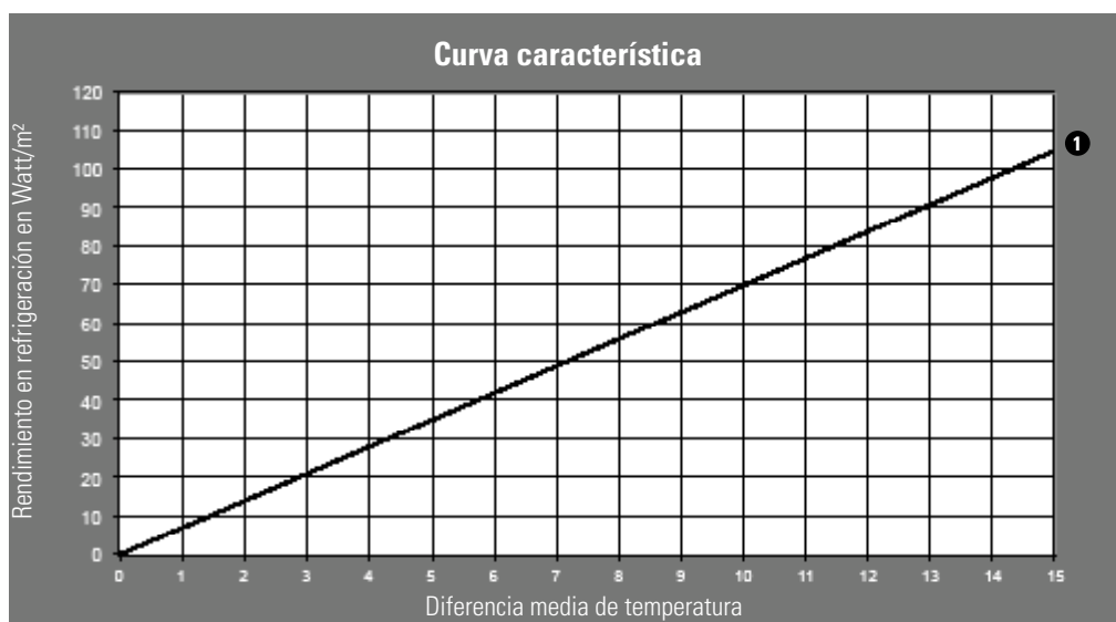
Curva característica
