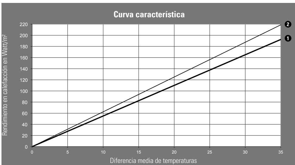
Curvas características
